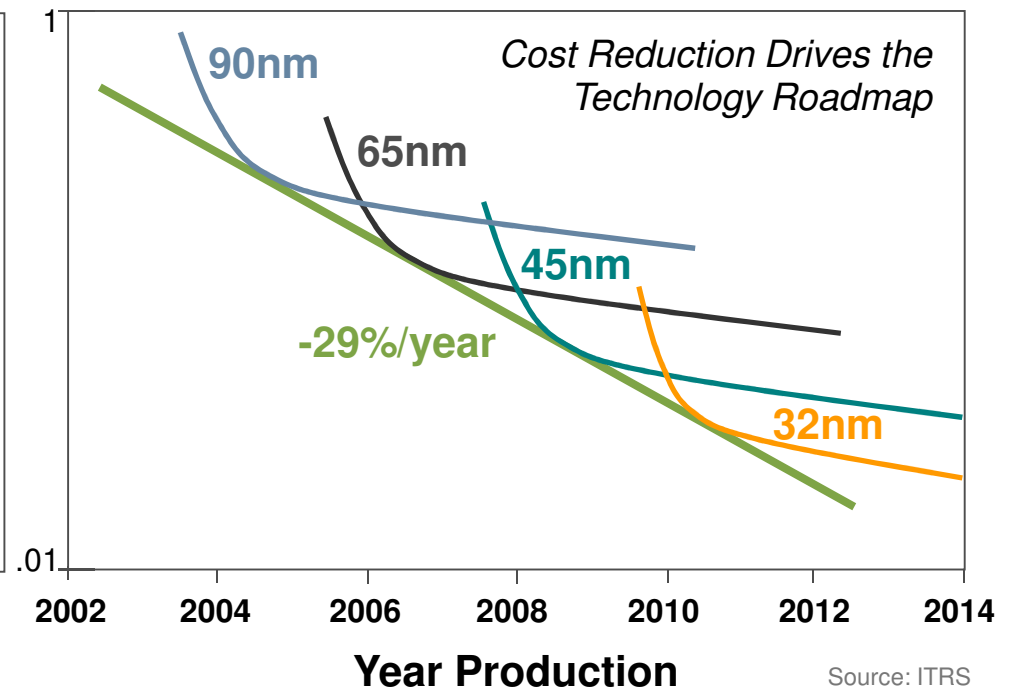
Relative Cost Per Gate (log scale)
